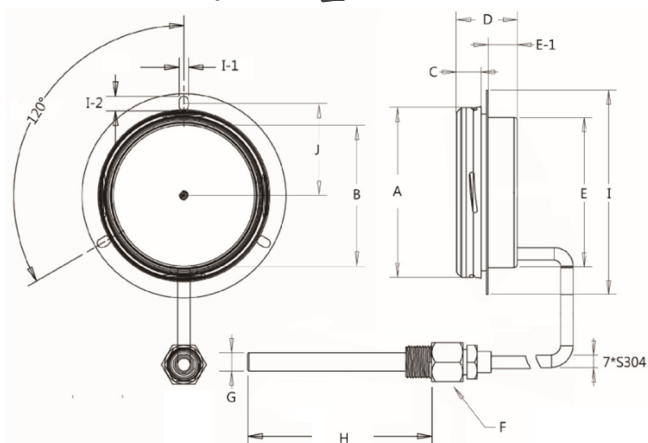
埋入 CF 型
